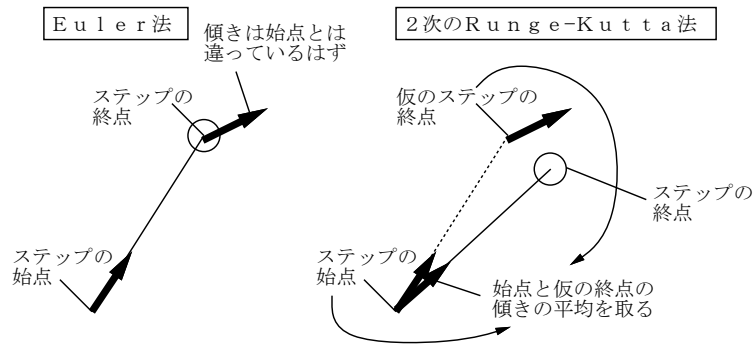
図 6: オイラー法と 2 次のルンゲ-クッタ法
